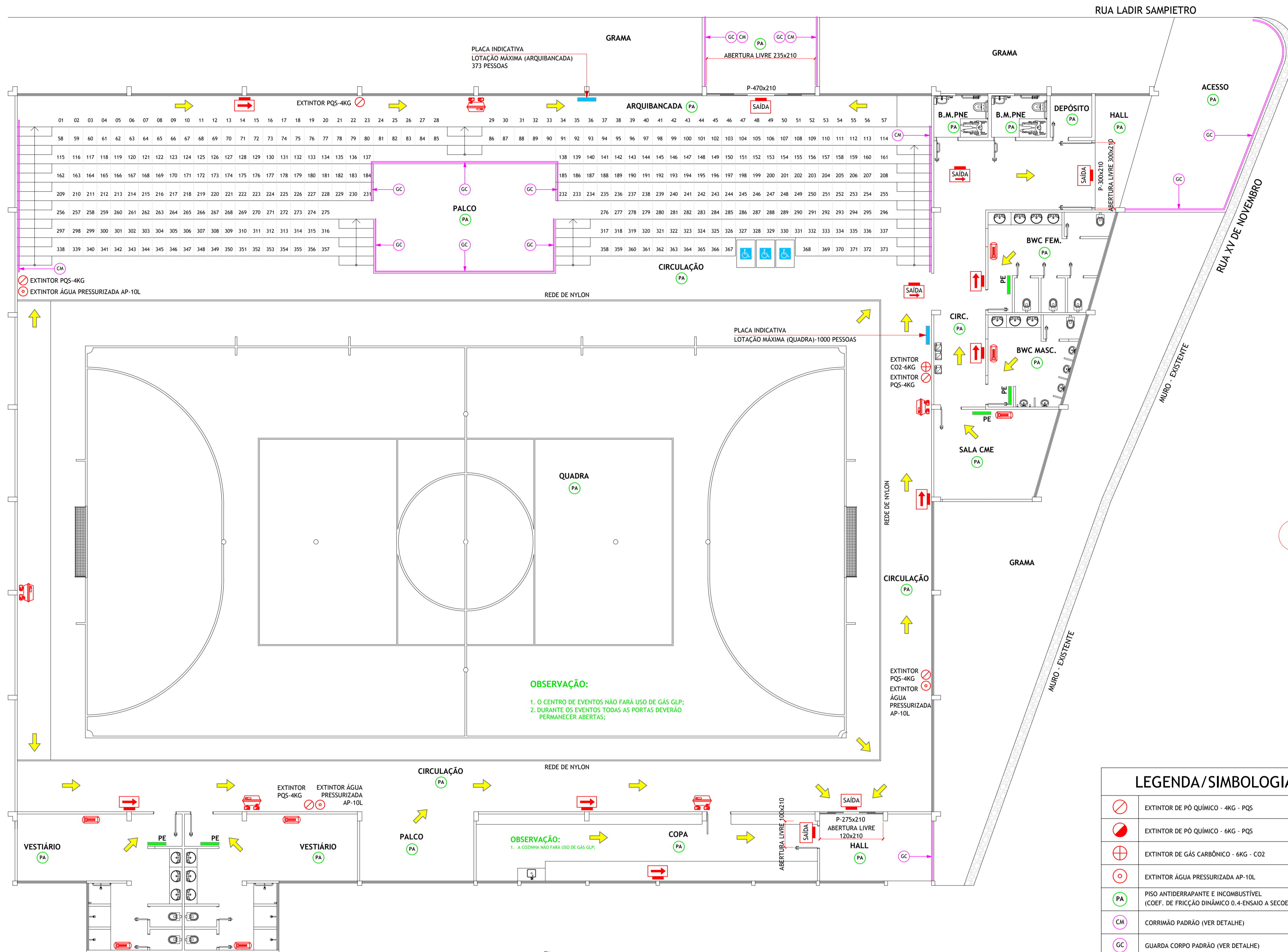
1 PLANTA BAIXA PAVTO. INFERIOR ÁREA: 1.512,56m 2 ESCALA: 1/100
