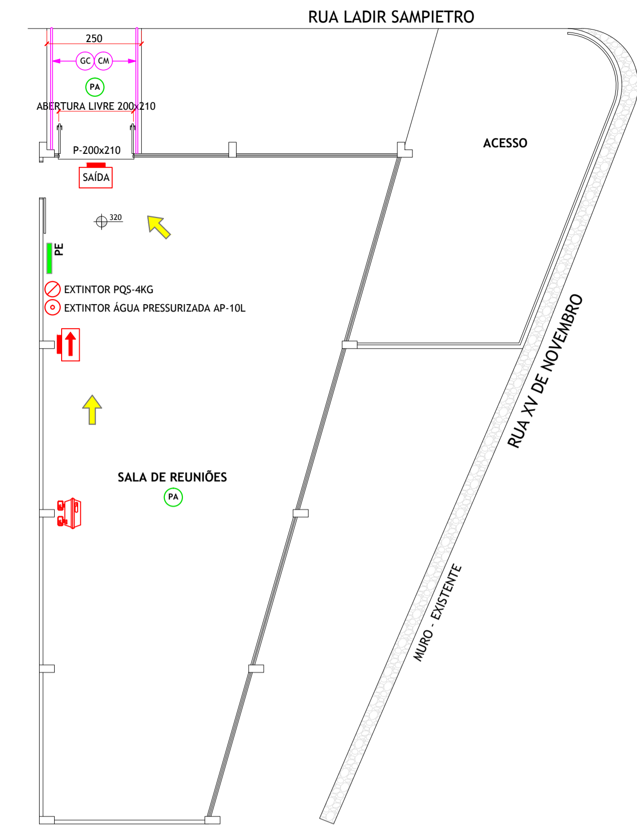
2 PLANTA BAIXA PAVTO. SUPERIOR ÁREA: 124,42m 2 ESCALA: 1/100
