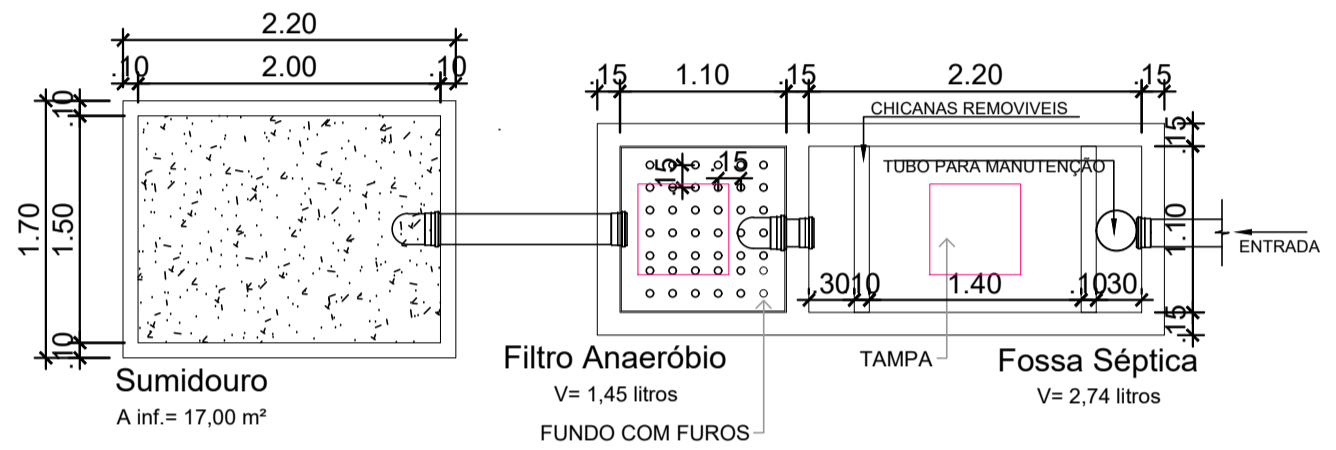
Detalhamento Sistema Tratamento ESC 1/50
