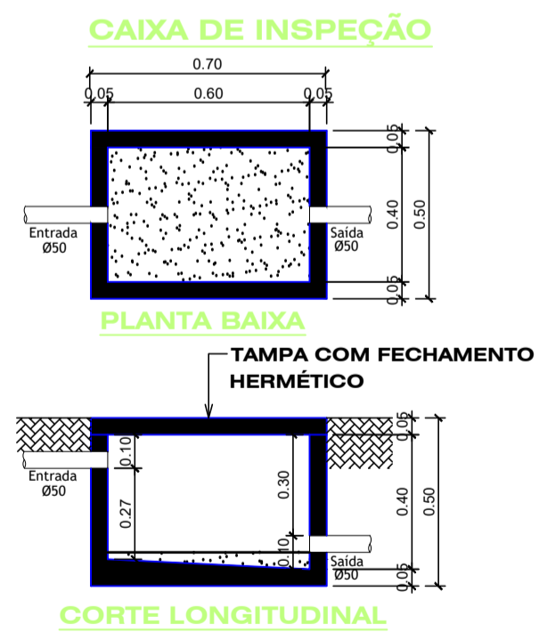
Detalhamento Sistema Tratamento ESC 1/50
