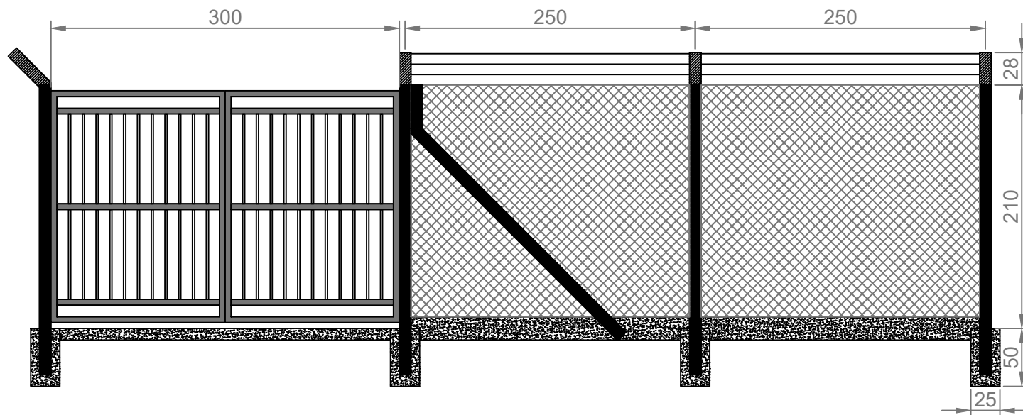
DETALHE - VISTA LATERAL - ALAMBRADO E PORTÃO
