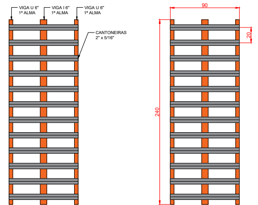
RAMPAS TRASEIRAS
