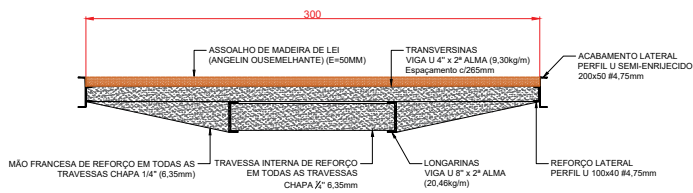
PERFIL TRANSVERSAL
