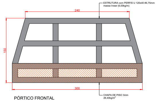
PÓRTICO FRONTAL
